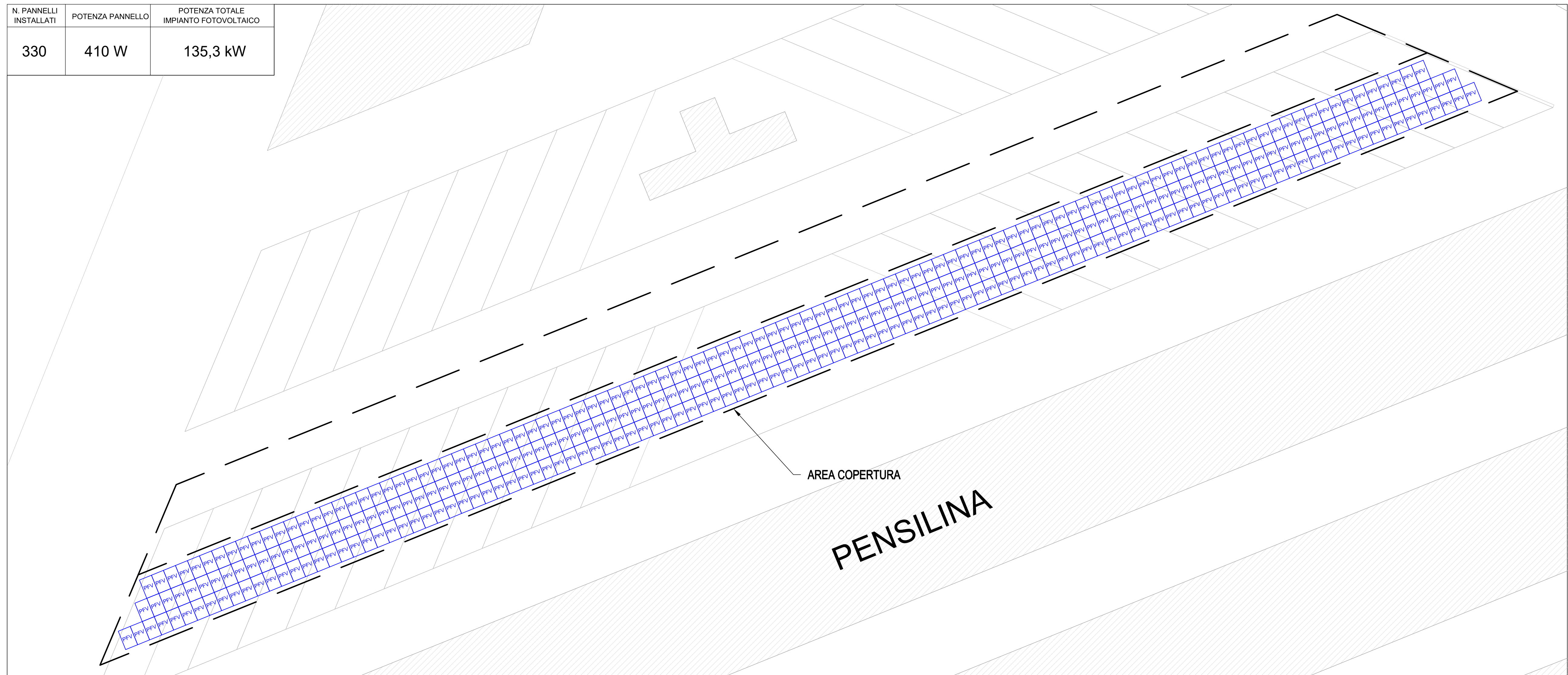
POSIZIONAMENTO PANNELLI FOTOVOLTAICI - SCALA 1:200
